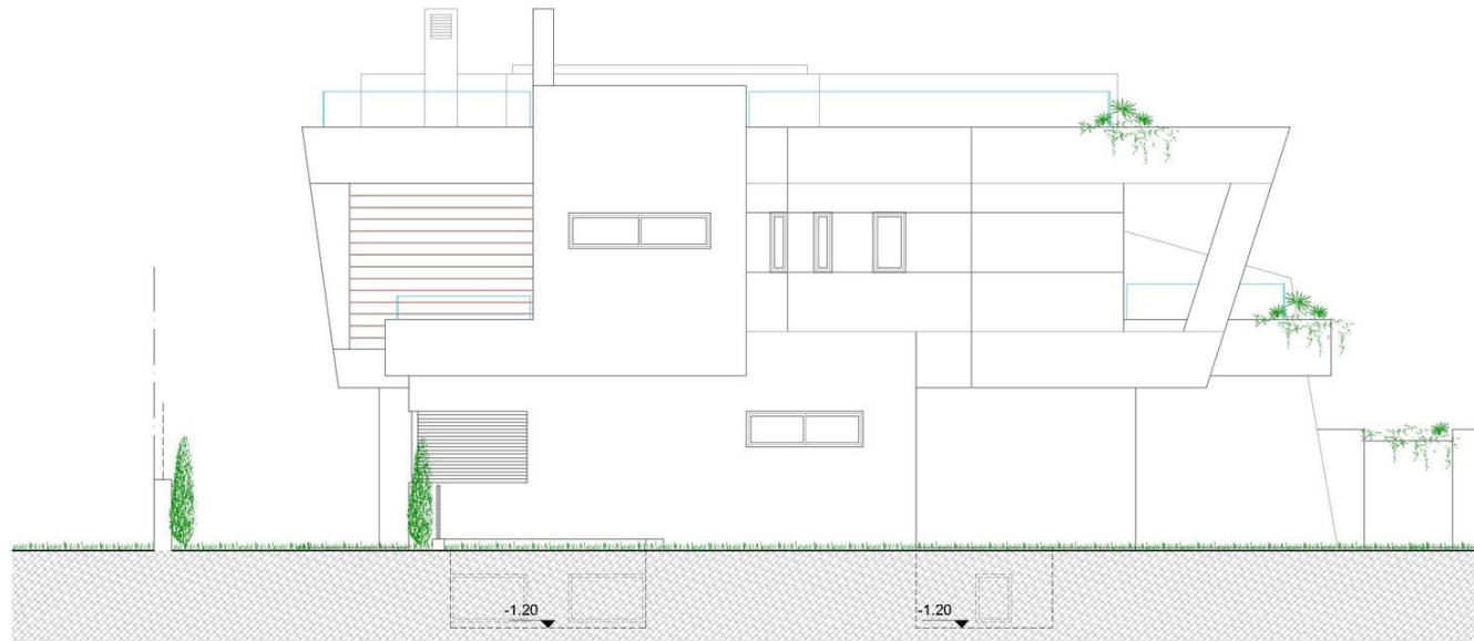
Alzado Lateral
