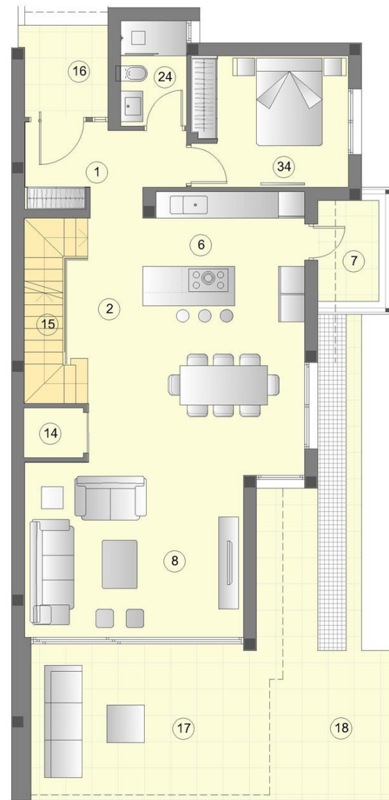
PLANTA BAJA
