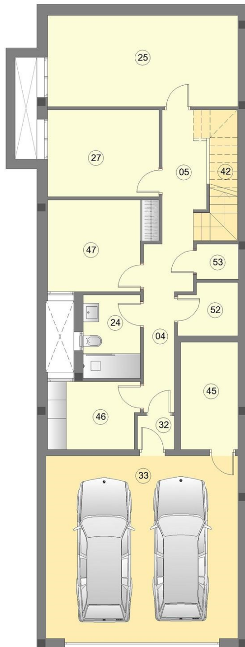
PLANTA SÓTANO
