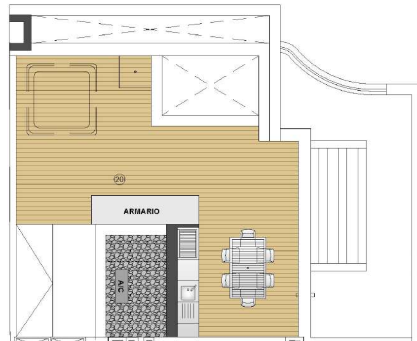
PLANTA SOLARIUM
