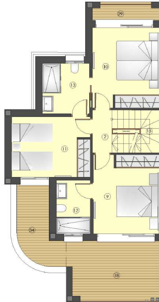
PLANTA PRIMERA
