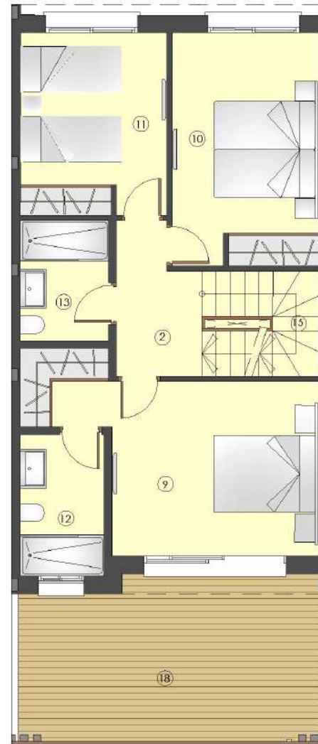
PLANTA PRIMERA
