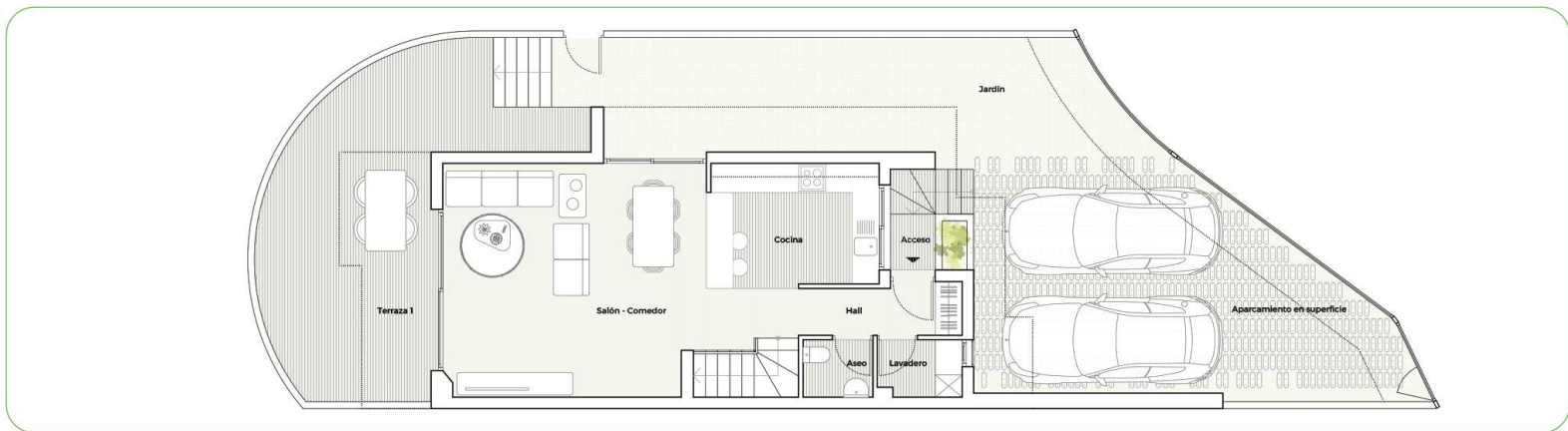
Planta baja
